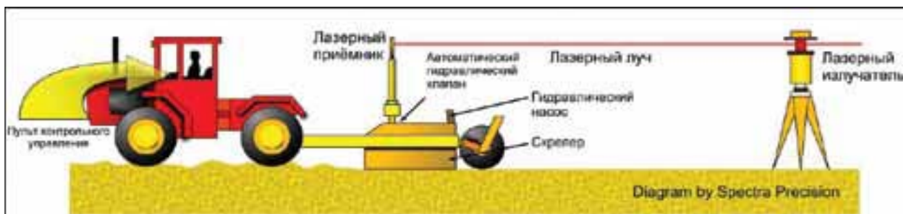
Рис. 2. Схема работы и компоненты лазерного планировщика
