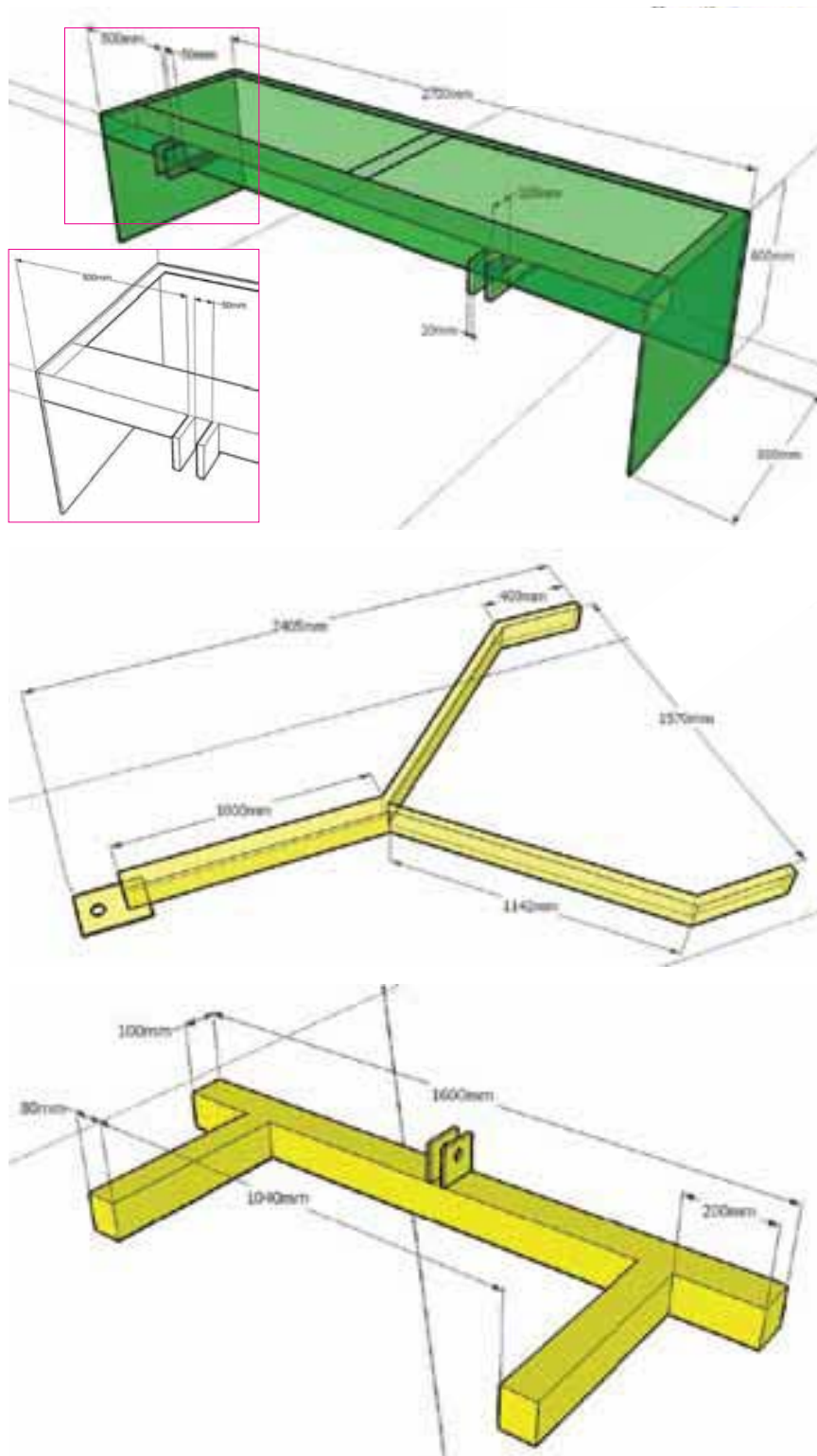
Рис. 7. Данные для изготовления бездонного ковша, прицепной рамы и оси для колес.
